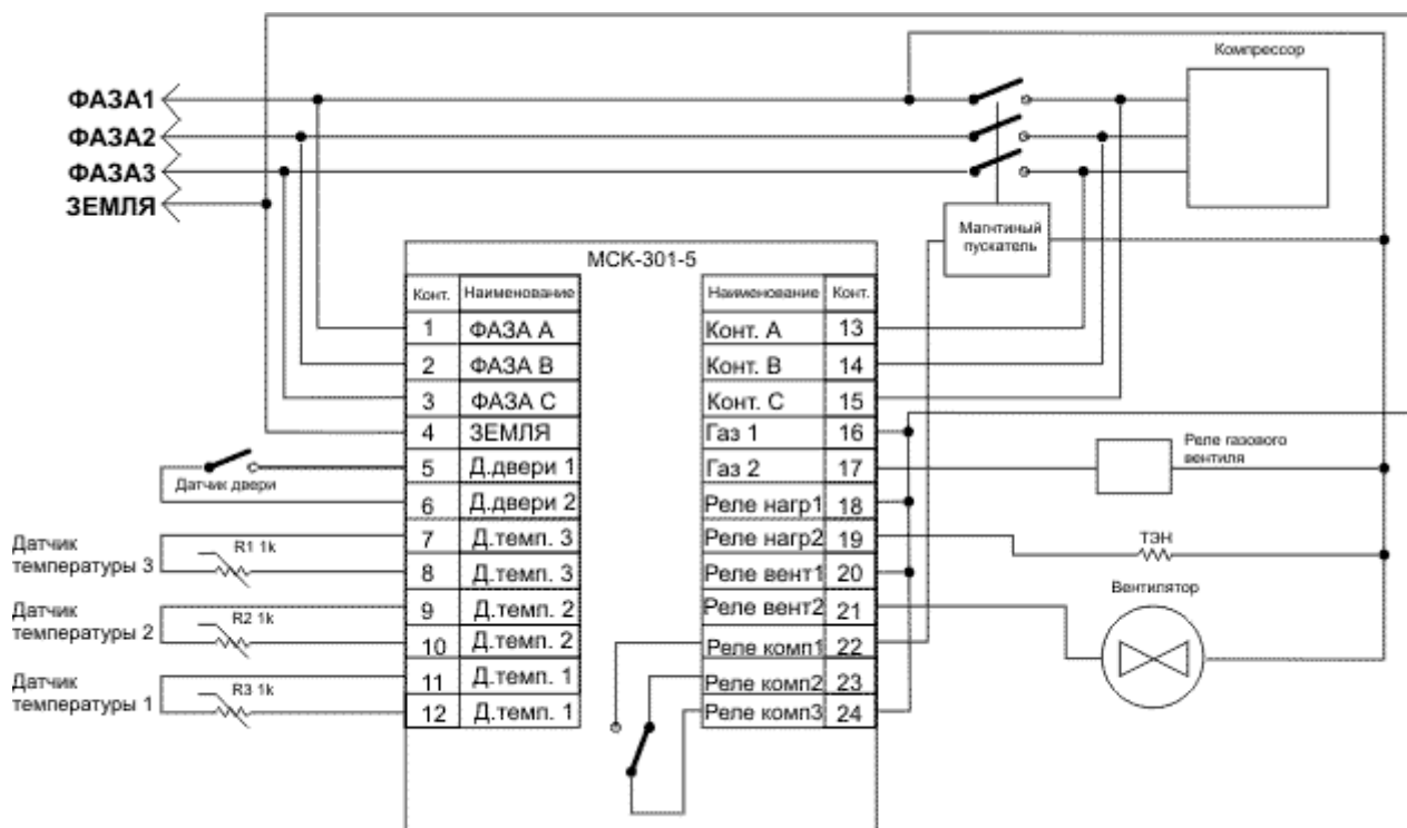
Рисунок 2. Схема подключения МСК-301-5 к трехфазной сети.
