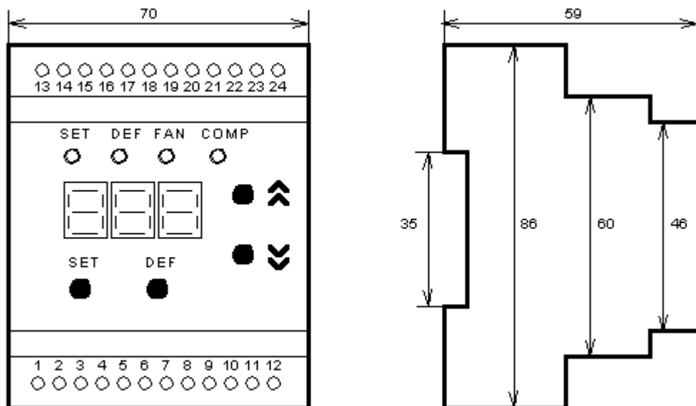
Рисунок 1. Лицевая панель, органы управления и габаритные размеры МСК-301-5.
